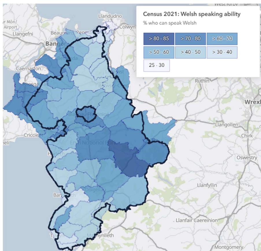
Ffigur B- 1-9: Dosbarthiad daearyddol siaradwyr Cymraeg yn Eryri
