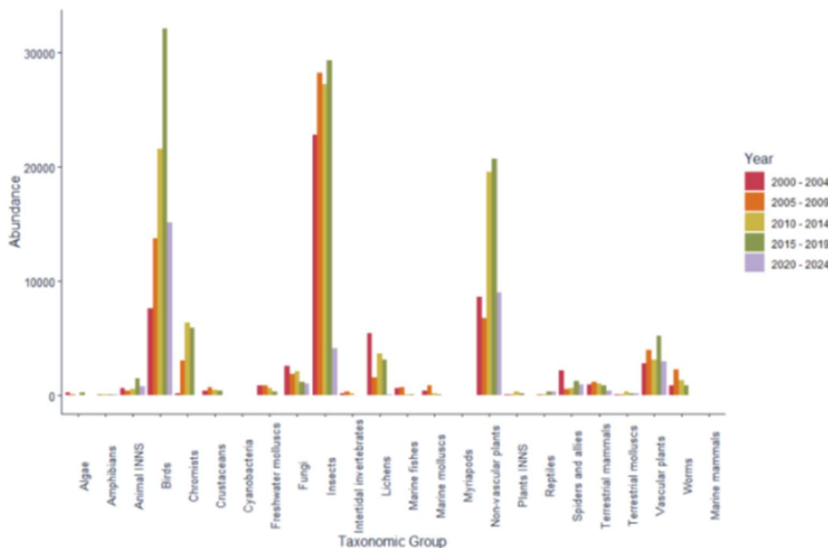
Ffigur B- 3 2 : Digonedd o ddata am yr holl rywogaethau o fewn APC Eryri ar gyfer cofnodion cyhoeddus 2000 – 2024 wedi'i rannu'n grwpiau tacsonomig (Llywodraeth Cymru, 2024)
