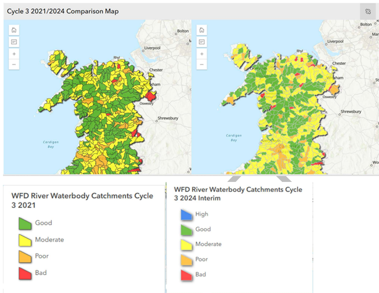
Ffigur B- 6 -5 : Statws cyflwr dalgylch corff dŵr y Gyfarwydddeb Fframwaith Dŵr 2021 vs 2024
