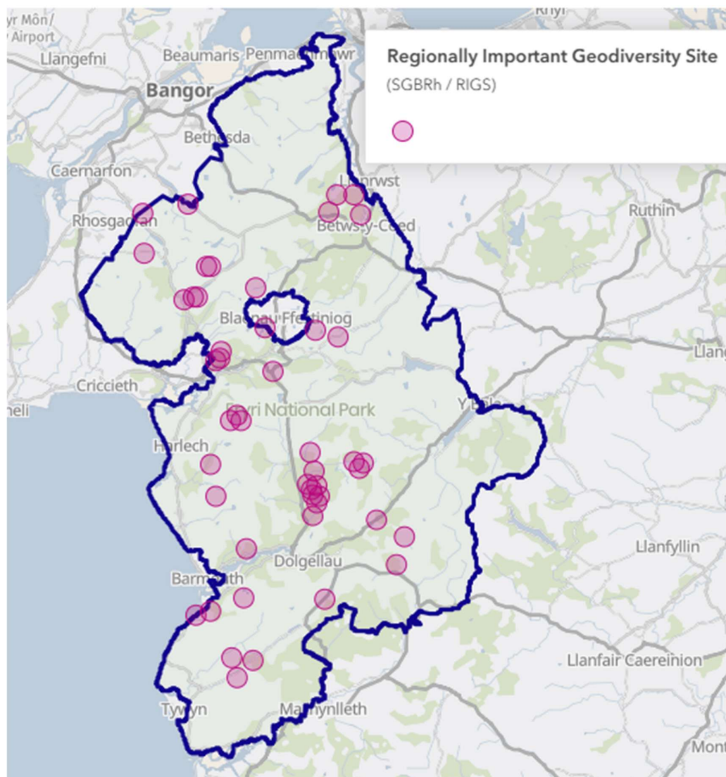
Ffigur B- 6 -3 : Safleoedd Geoamrywiaeth Pwysig yn Rhanbarthol yn Eryri
