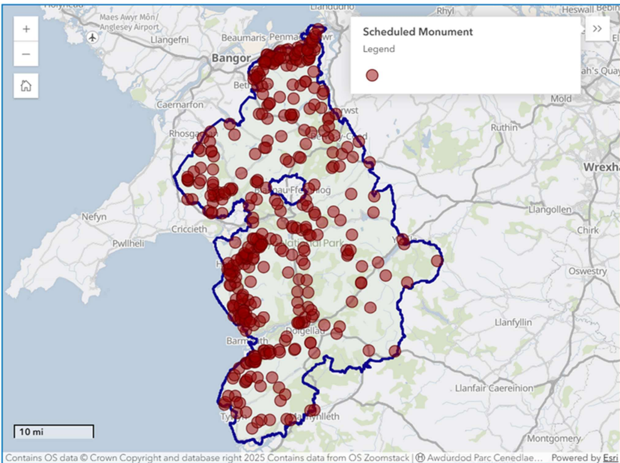
Ffigur B- 8 -1 : Henebion Rhestredig yn Eryri
