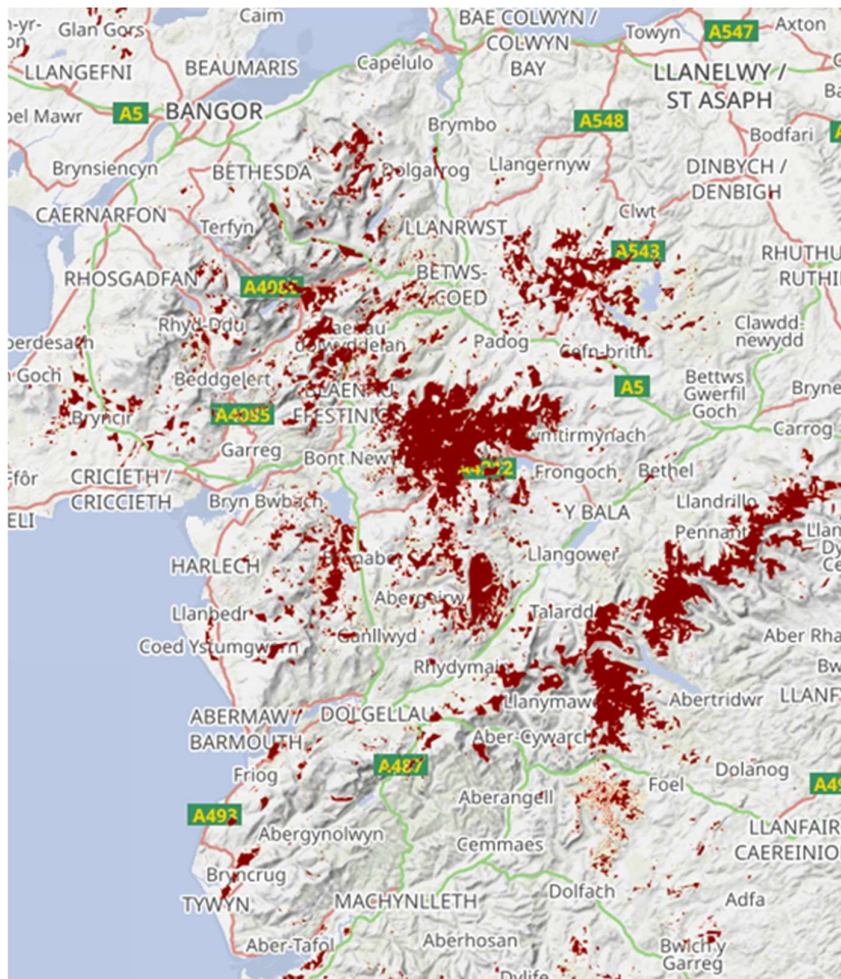
Ffigur B- 6 -2 : Mawndiroedd Cymru
