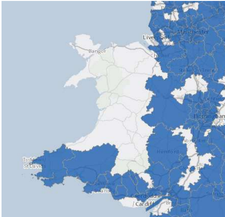
Ffigur B- 5 -4 : Ardaloedd Rheoli Ansawdd Aer Cymru
